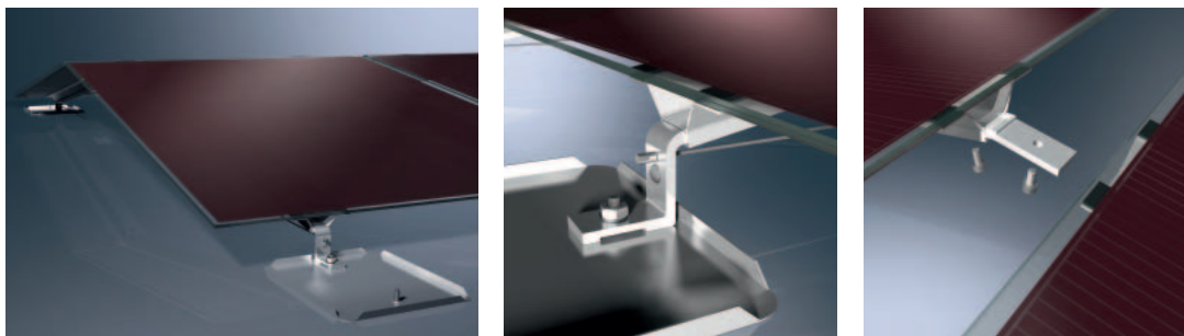
Das Schüco Montagesystem MSE 100 Flachdach Ost/West bildet selbsttragende, dachförmige statische Einheiten
